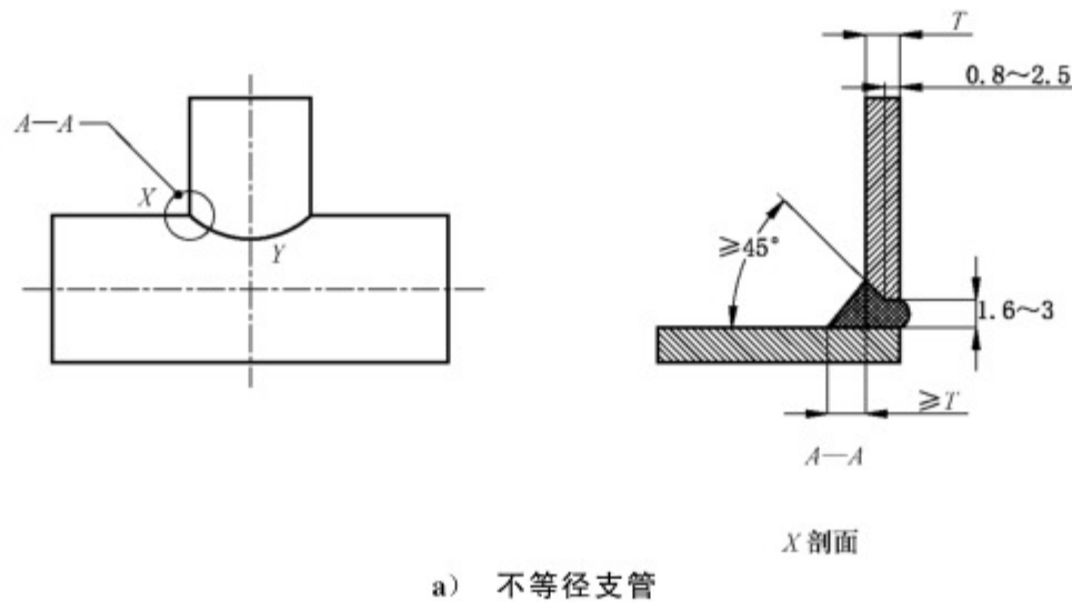
图 7 三通支管焊接
