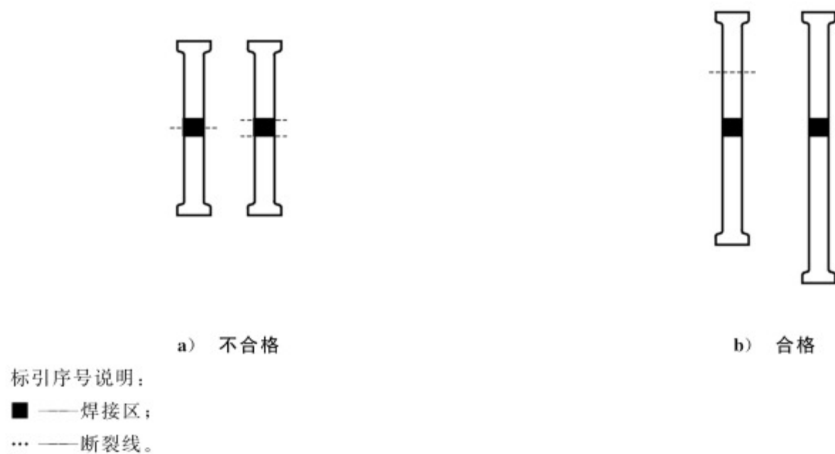
图 B.2 拉伸后试样合格判定示意
