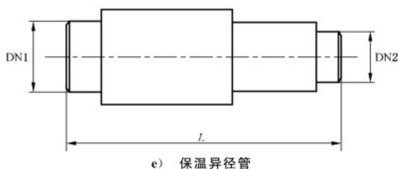
图 10 保温管件主要尺寸允许偏差示意 (续)
