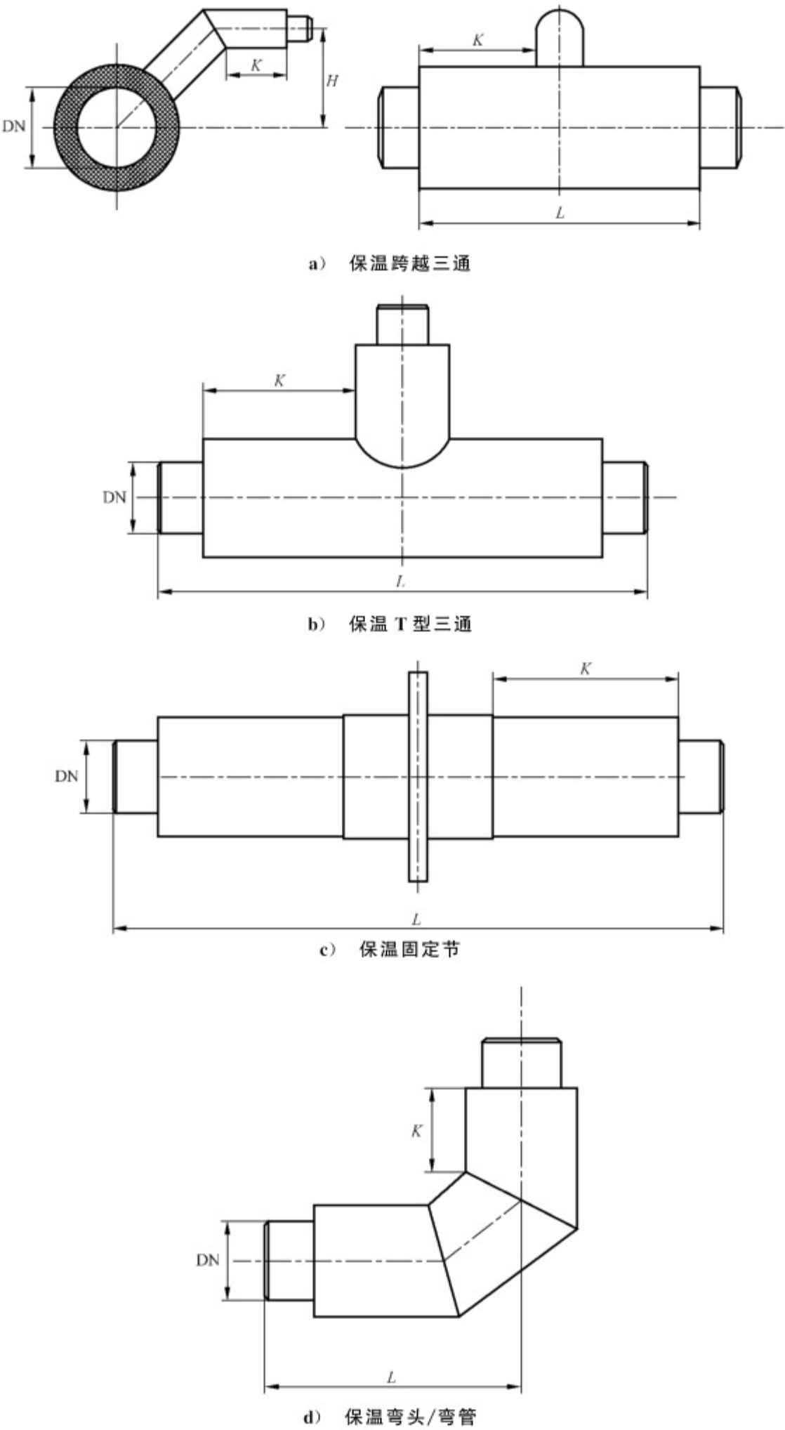
图 10 保温管件主要尺寸允许偏差示意
